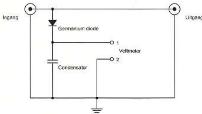
Figuur 1. Eenvoudige vermogensmeter: Sluit de zender aan op de ingang. Plaats aan de uitgang een geschikte antenne of dummyload. Via de germanium diode (lagere spanningsval) wordt de condensator (1 nF - 1mF) tot de piekspanning van het HF-signaal geladen. Deze spanning kan vervolgens met een hoogohmige voltmeter bepaald worden. Bij een bekende belasting en spanningsval over de diode, is dan in principe ook het vermogen van de zender bekend.
